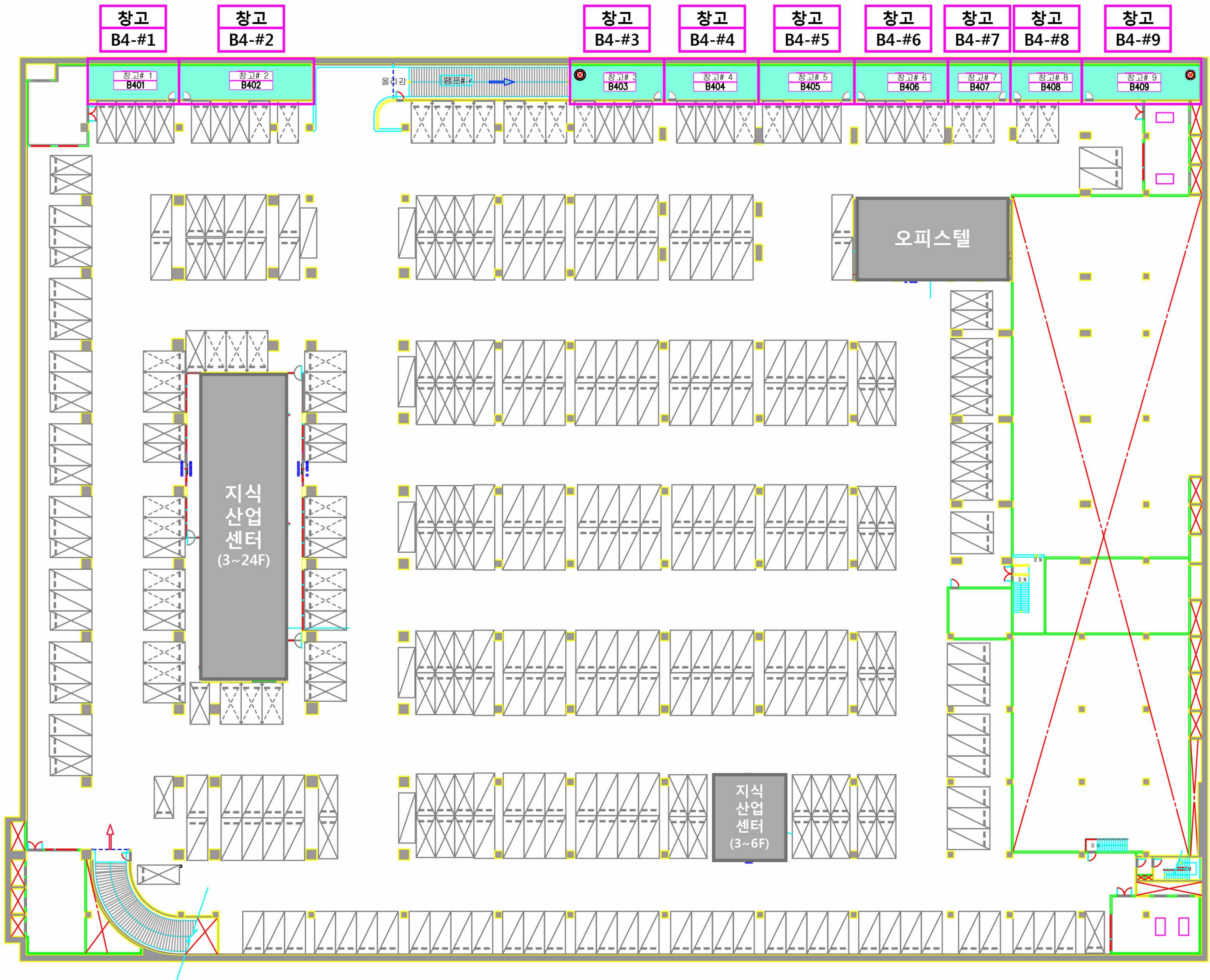
■ 지하4층 평면도
