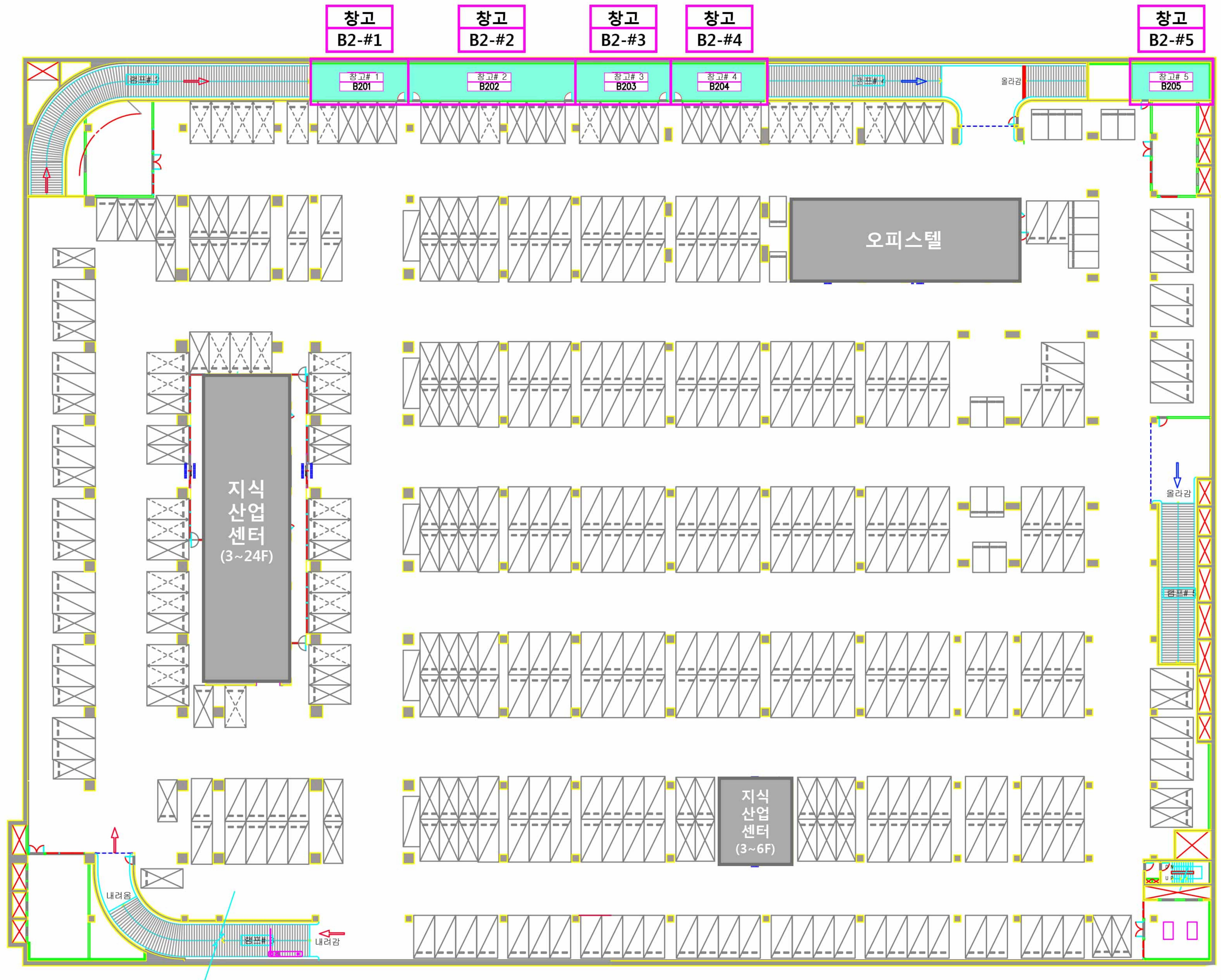
■ 지하2층 평면도
